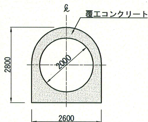
《覆工コンクリート断面図》
